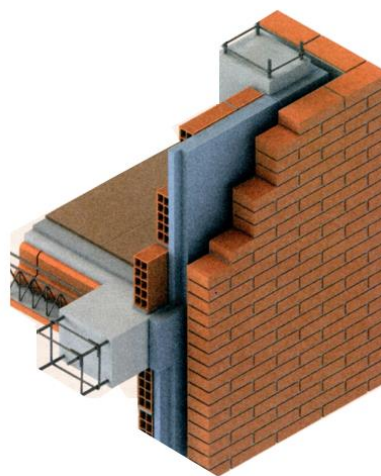
DOPPIA PARETE CON INTERCAPEDINE D'ARIA
